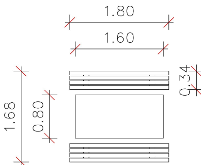
Stół do szachów i chińczyka do wkopania nr kat. 12.5.04
