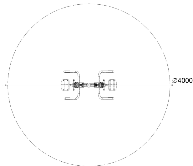
Wyciąg górny nr kat. 14.1.06
