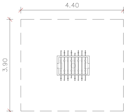
Stół do gry w piłkarzyki nr kat. 12.6
